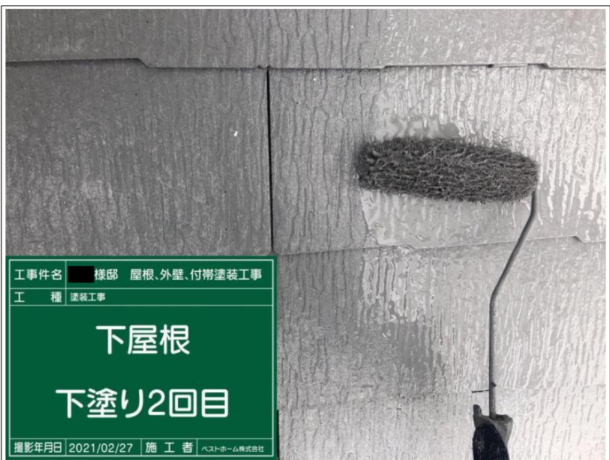
工事件名 ■ 棟邸 屋根、外壁、付帯塗装工事 工 種 塗装工事 下屋根 下塗り2回目 撮影年月日 2021/02/27 施 工 者 ヘスト京一ム株式会社
