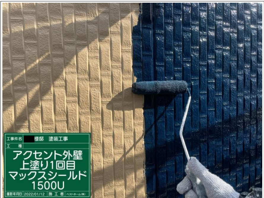
工事件名 棟邸 塗装工事 工 種 アクセント外壁 上塗り1回目 マックスシールド 1500U 撮影年月日 2022/01/12 施 工 者 ベストホーム(株)
