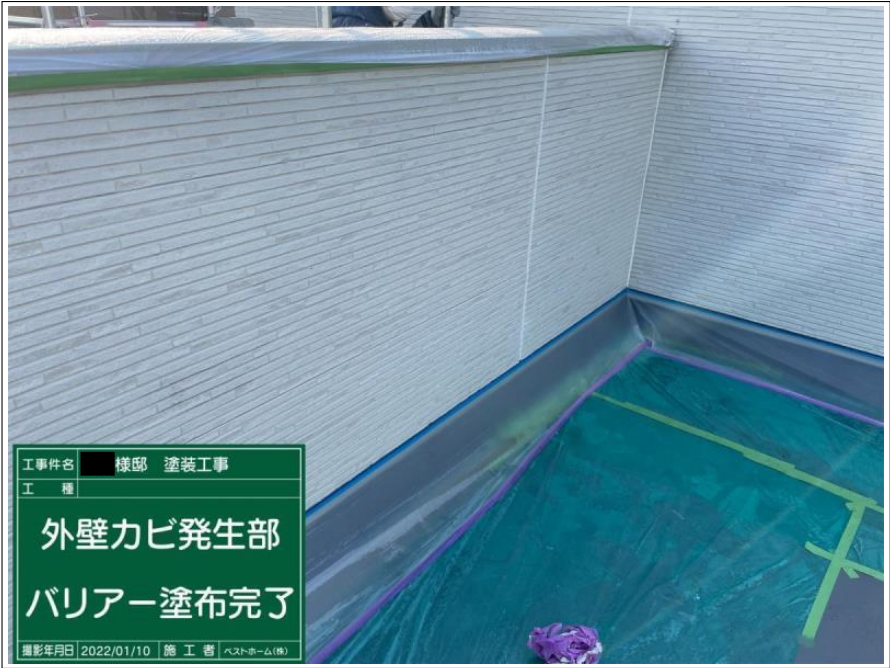
工事件名 様邸 塗装工事 工 種 外壁カビ発生部 バリアー塗布 撮影年月日 2022/01/10 施 工 者 ベストホーム(株)
