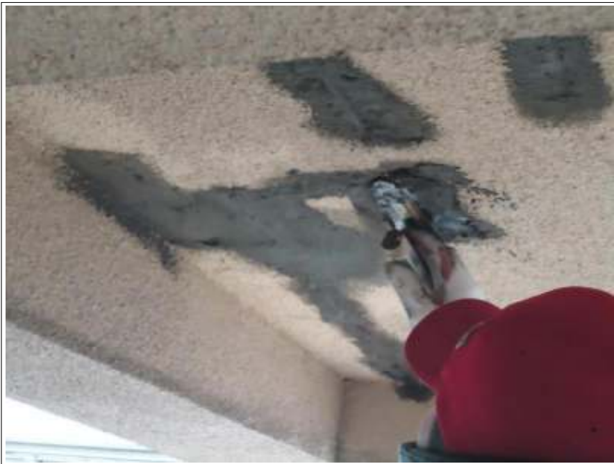
爆裂部 モルタル補修施工中
