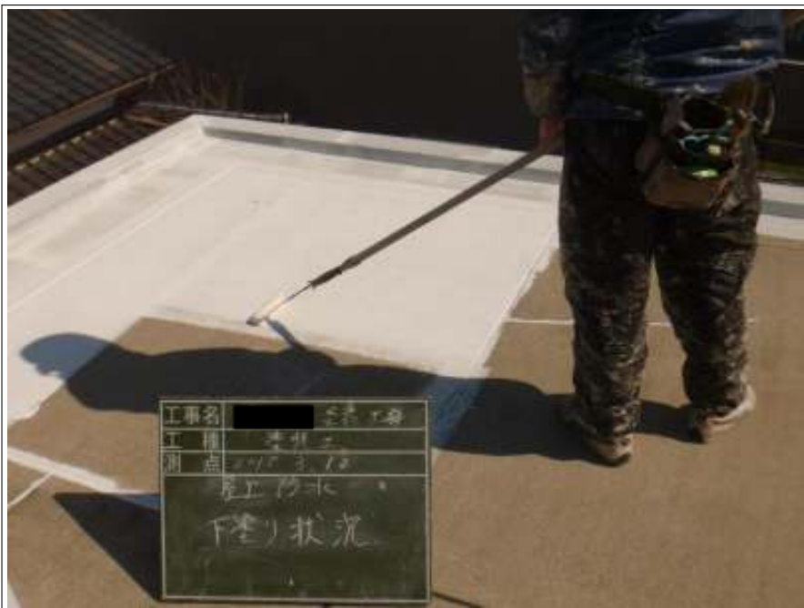
屋上防水下塗り施工中
